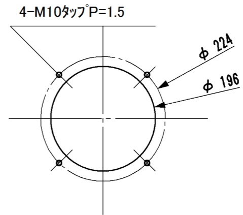
旋回フランジ取付穴
